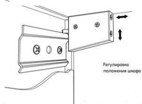
Схема крепления и регулирования направляющих (рис.8)
