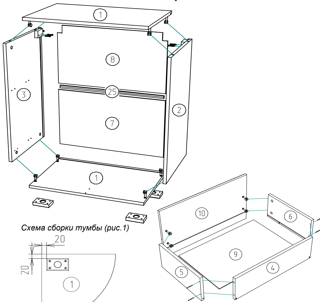
Схема сборки ящика (рис.2)
