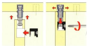
Схема установки эксцентриковой стяжки (рис.4)
