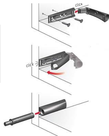
Схема установки толкателя(рис.11)
